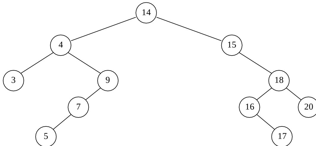
Fig 13.4: Inorder: 3 4 5 7 9 14 15 16 17 18 20
